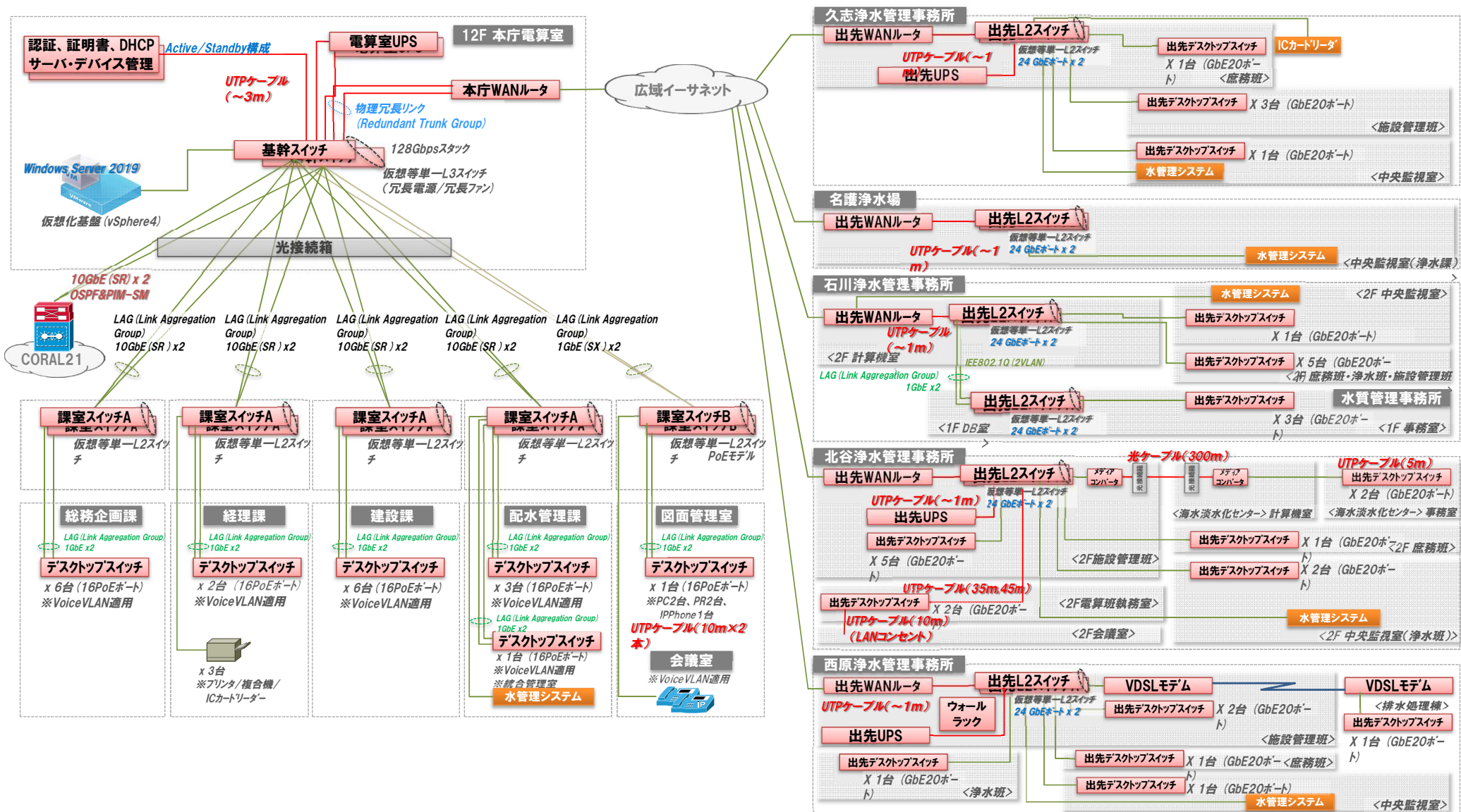
全体ネットワーク構成図
